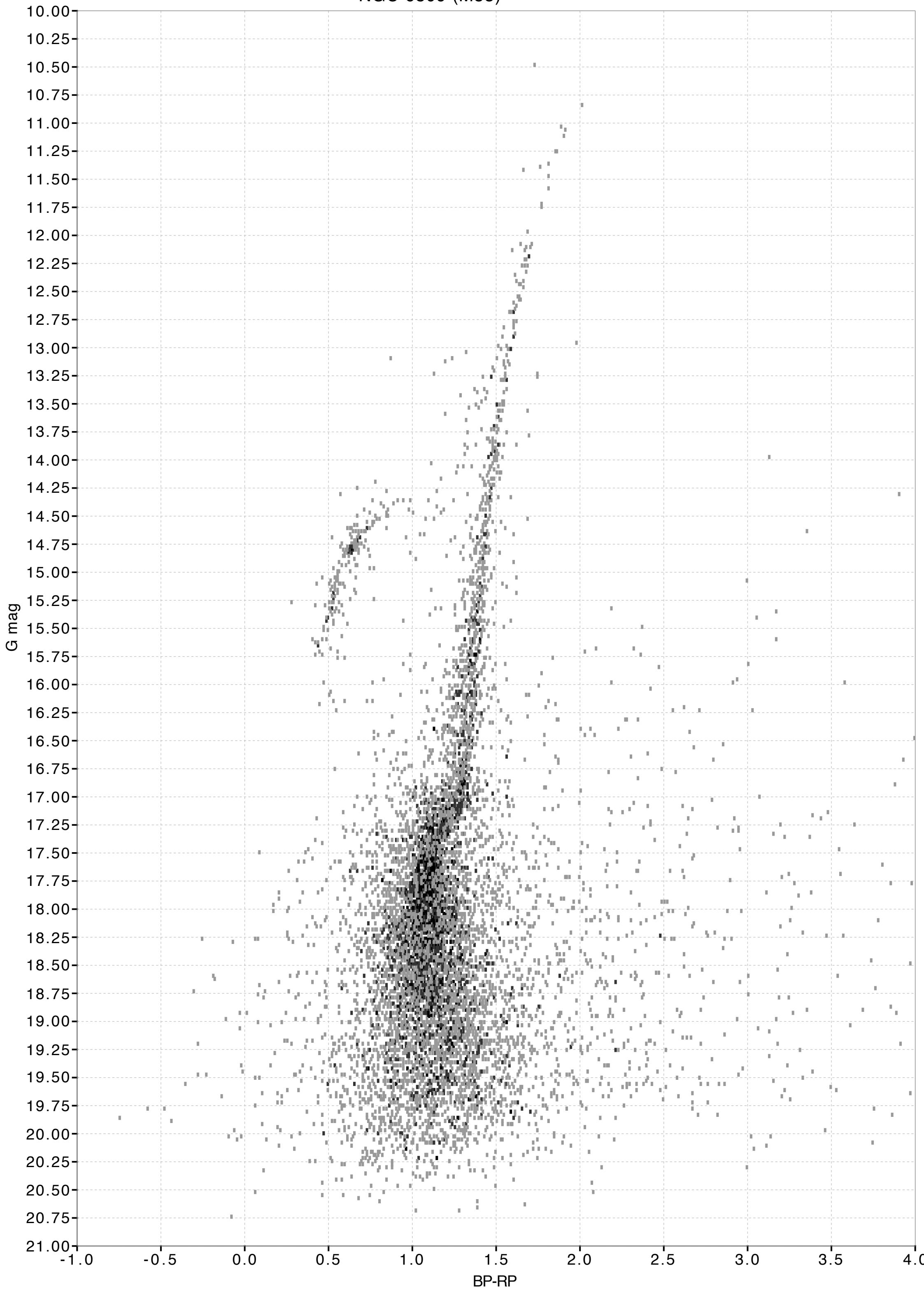
NGC 6809 (M55)
