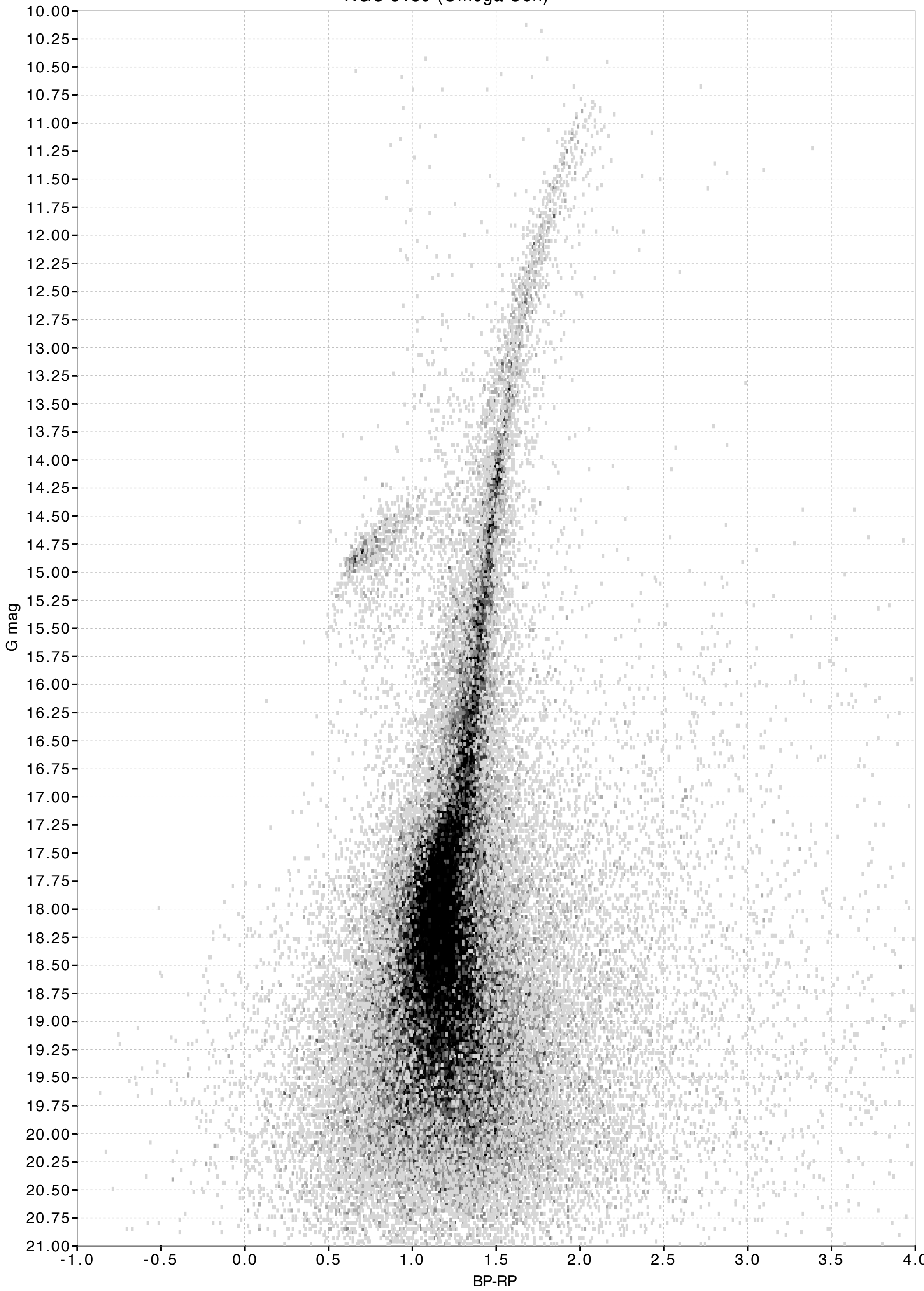
NGC 5139 (Omega Cen)
